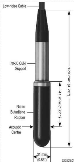
Хидрофон "Brüel&Kjær" тип 8104
